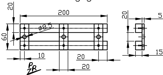
Guides de perçage poutre Beam drilling guides
