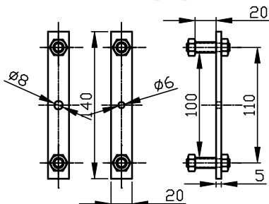
Guides de perçage poutre Beam drilling guides
