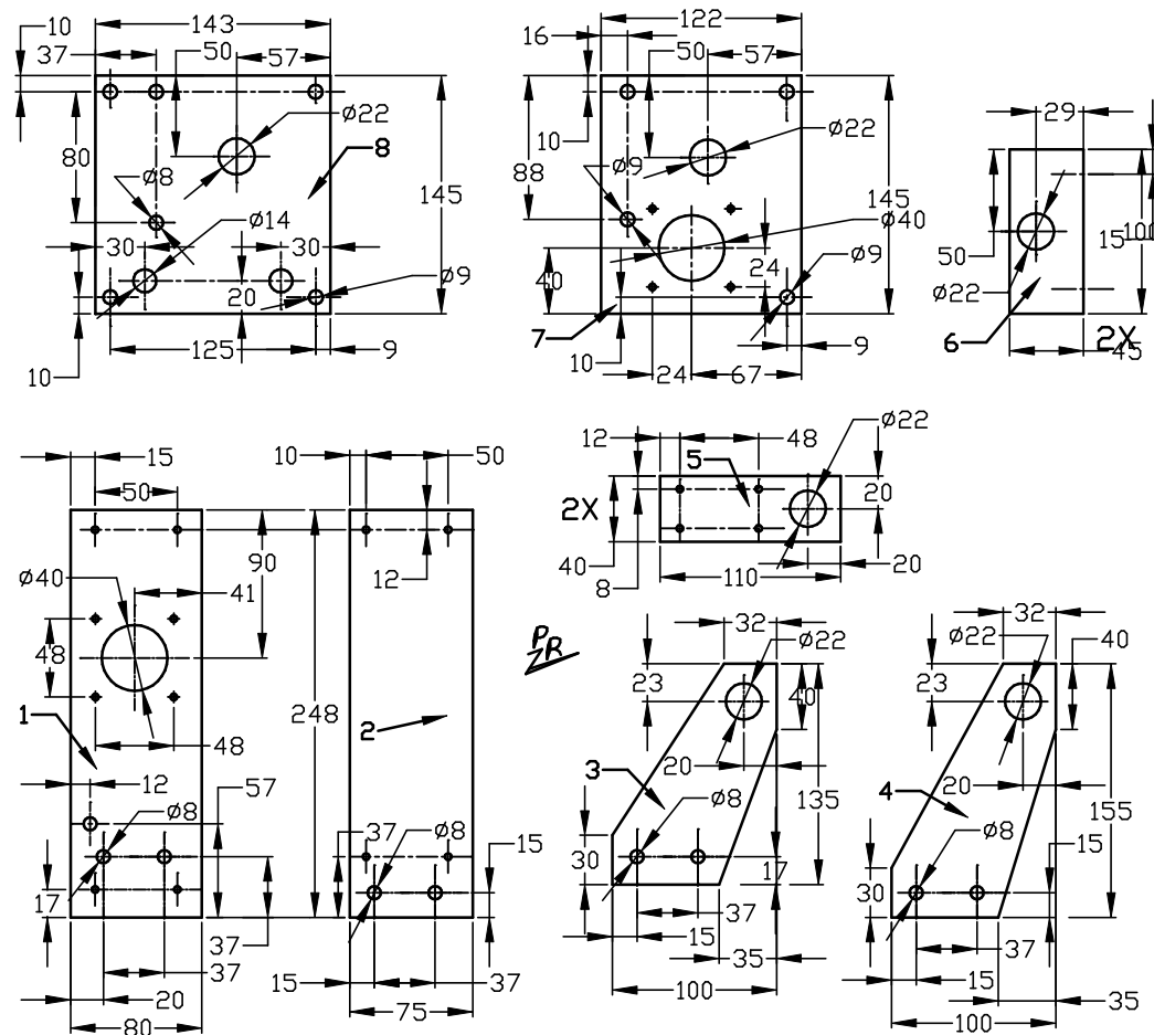
Plates designed for NEMA 23 motor size / Plaques dessinées pour un moteur taille NEMA 23 (57 x57)
